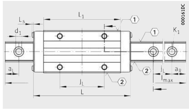
KUVE...-B-HL, KUVE...-B-SL, KUVE...-B-SNL View X rotated 90°
