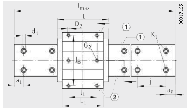
KUVE...-W, KUVE...-WL View X rotated 90°
