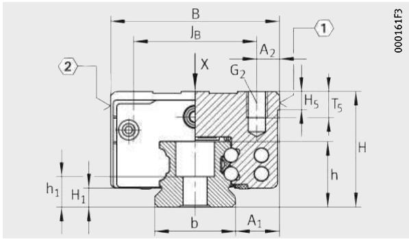
KUVE...-B-ES
