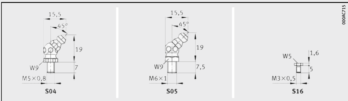
Lubrication connectors 4)
