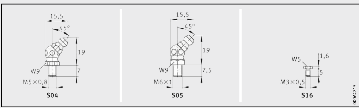
Lubrication connectors 3)
