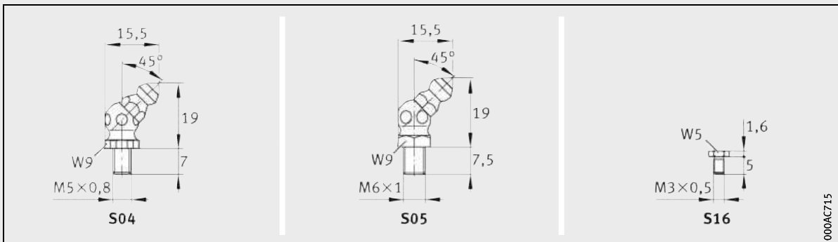
Lubrication connectors 4)
