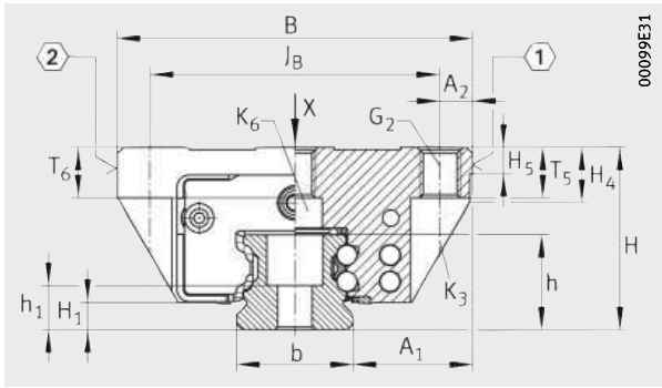
KUVE25-B-HS, KUVE25-B-E-HS, KUVE25-B-N-HS
