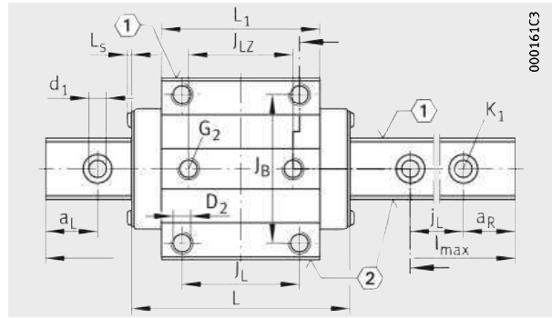
KUVE...-B, KUVE...-B-L, KUVE...-B-N, KUVE...-B-NL View X rotated 90°
