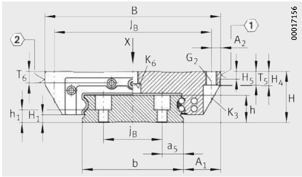
KUVE...-W, KUVE...-WL
