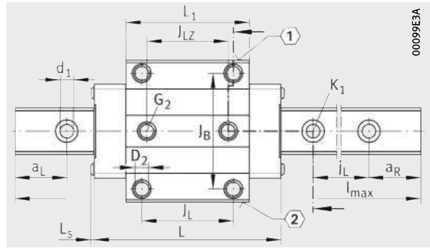
KUVE25-B-HS, KUVE25-B-E-HS, KUVE25-B-N-HS View X rotated 90°
