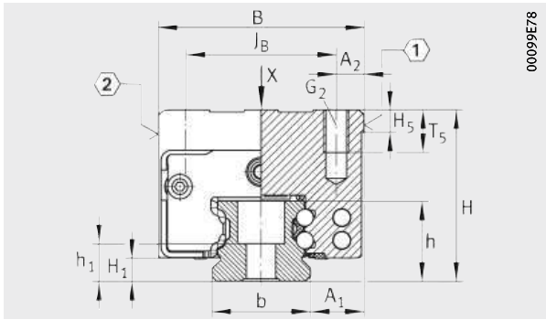
KUVE25-B-ES-HS, KUVE25-B-H-HS, KUVE25-B-S-HS, KUVE25-B-SN-HS
