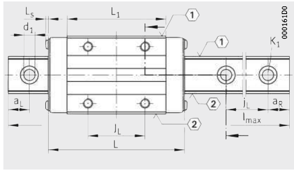
KUVE...-B-H, KUVE...-B-S, KUVE...-B-SN View X rotated 90°
