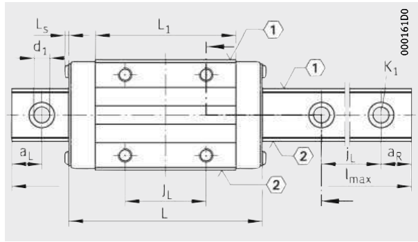
KUVE...-B-ES View X rotated 90°
