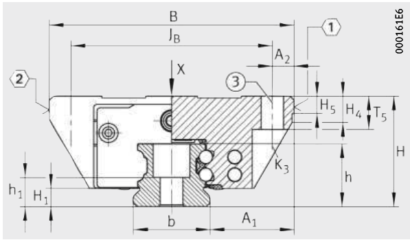
KUVE...-B-E
