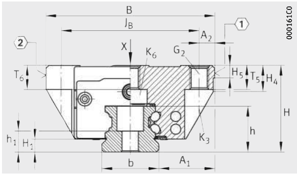
KUVE...-B, KUVE...-B-L, KUVE...-B-N, KUVE...-B-NL
