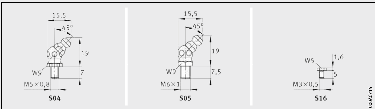
Lubrication connectors 5)
