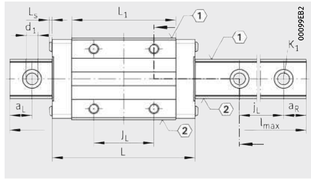
KUVE25-B-ES-HS, KUVE25-B-H-HS, KUVE25-B-S-HS, KUVE25-B-SN-HS View X rotated 90°
