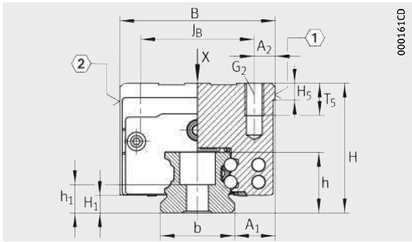
KUVE...-B-H, KUVE...-B-S, KUVE...-B-SN
