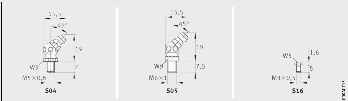
Lubrication connectors 3)
