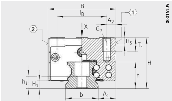
KUVE...-B-HL, KUVE...-B-SL, KUVE...-B-SNL
